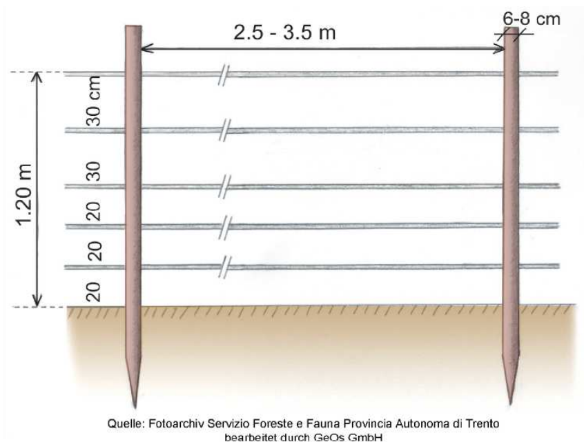
Abb. 12. In gefährdeten Regionen setzen Imker bei der Schadenverhütung auf ein erprobtes Elektrozaunsystem. Eine stabile Bauweise und gute Wartung sind Voraussetzung für einen wirkungsvollen Schutz.
