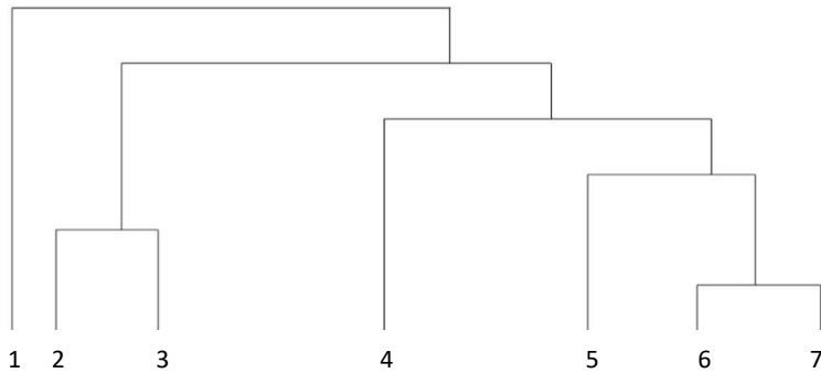
Abbildung 5: Dendrogramm der Klassifikation mit TWINSpan.
