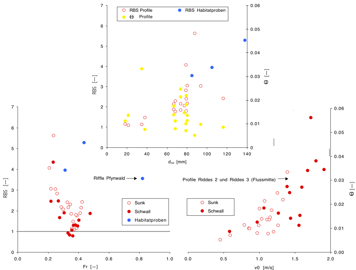
Abbildung 14. Beziehung zwischen verschiedenen hydraulischen Parametern aus Querprofilen und Mesohabitaten der Rhone im Winter 2002. Linkes Bild: Relative Bettstabilität RBS und Froudezahl Fr . Rechtes Bild: Dimensionslose Sohlenschubspannung \Theta und Oberflächenströmung v_0 . Sunkwerte sind gemessen, Schwallwerte berechnet mittels HEC-RAS (LCH, 2002). Mittleres Bild oben: RBS , \Theta und mittlerer Korndurchmesser d_{50} . Nur Werte bei Sunk aufgetragen.
