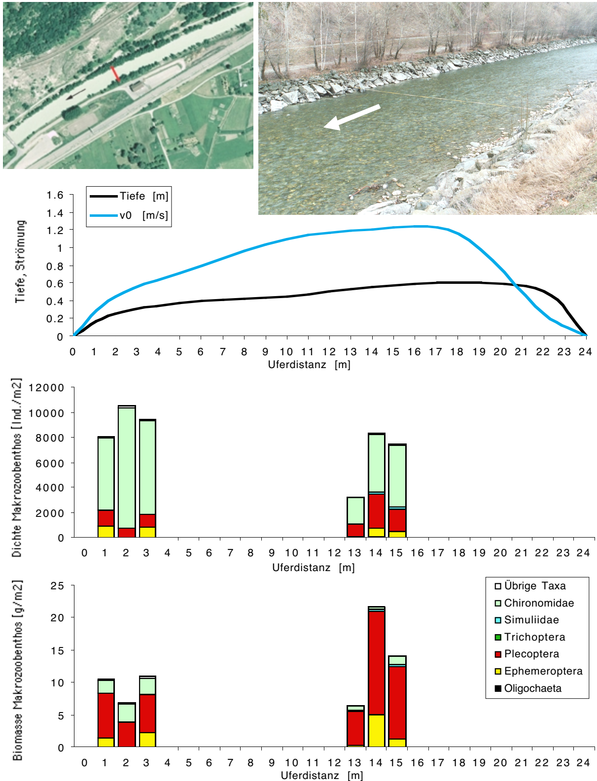
Abbildung 26. Das Makrozoobenthos im Querprofil der Rhone bei Brig. Von oben nach unten: Luftaufnahme bei hohem Wasserstand im Sommer 1999 oder 2000 mit der Lage des Querprofils (roter Balken) und Ansicht des Profils zum Zeitpunkt der Aufnahmen; Wassertiefen und Oberflächenströmung v0 über das Profil bei tiefem Abfluss am 3.3.2002; Abundanz (Individuendichte) und Biomasse (Frischgewicht) des Makrozoobenthos in Einzelproben über das Profil am 3.3.2002, aufgeteilt nach den wichtigsten vertretenen, systematischen Gruppen. Darstellungen der Querprofile in Fliessrichtung betrachtet. Luftbild: Aufnahme "Swissimage", © Office fédéral de topographie (DV023268).
