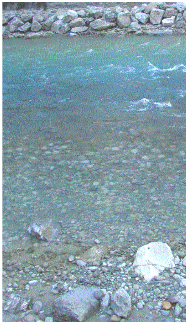
Abbildung 23. Makroalgen-Bewuchs in der Rhone im Spätwinter (März). Bild links oben: Riffle in der Restwasserstrecke von Iles Falcon mit dichtem Kieselalgenbelag und fädigen Grünalgen ( Cladophora sp.) bis zur Uferlinie. Bild links unten: Blockwurf in der Schwallstrecke von Riddes 1 mit dichtem Bewuchs von Cladophora sp., teils über der aktuellen Wasserlinie. Bilder rechts: Schwallstrecke bei Chippis mit Bewuchs der fädigen Grünalge Ulothrix sp. an und teilweise über der aktuellen Wasserlinie (oben); weiter flussaufwärts folgen bei genügend flachem Ufer zuerst eine weitgehend bewuchsfreie Zone und danach ein brauner Streifen mit dichteren Kieselalgenbelägen (unten).
