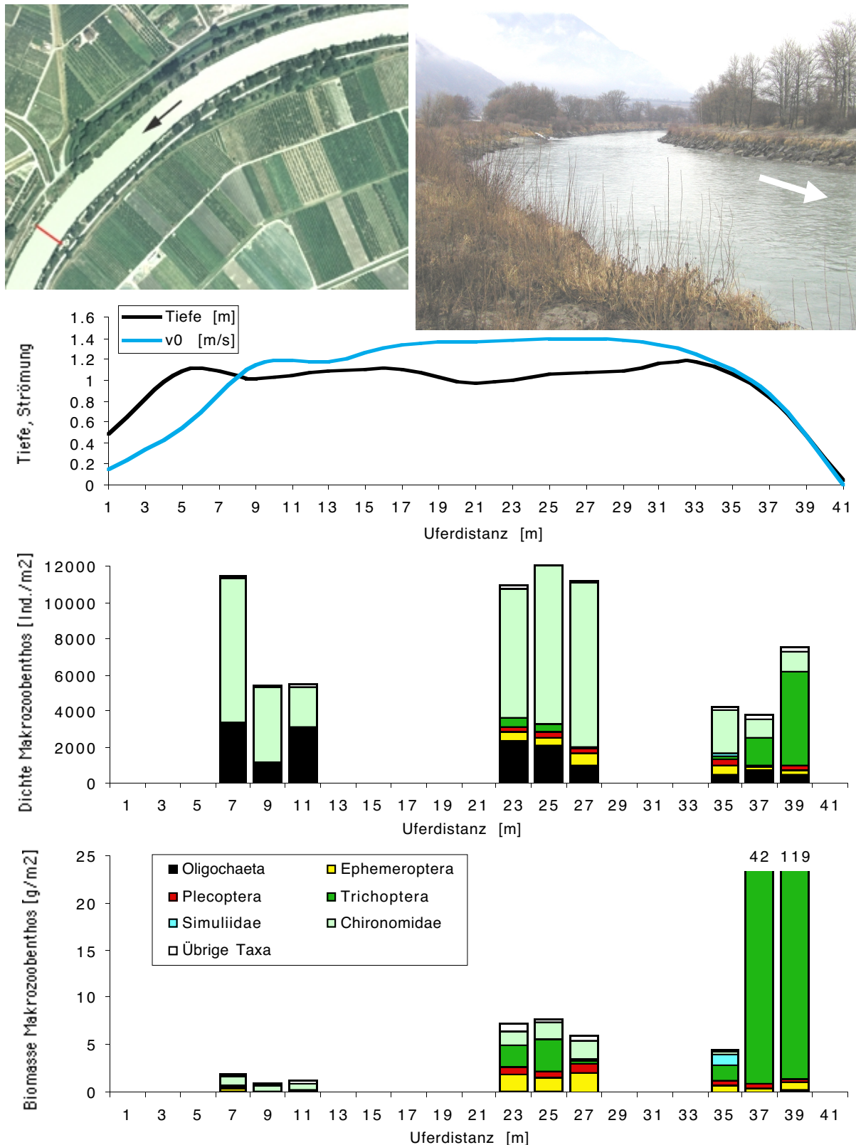
Abbildung 30. Das Makrozoobenthos im Querprofil der Rhone bei Riddes 3. Von oben nach unten: Luftaufnahme bei hohem Wasserstand im Sommer 1999 oder 2000 mit der Lage des Querprofils (roter Balken) und Ansicht des Profils zum Zeitpunkt der Aufnahmen; Wassertiefen und Oberflächenströmung v_0 über das Profil bei tiefem Abfluss am 2.3.2002; Abundanz (Individuendichte) und Biomasse (Frischgewicht) des Makrozoobenthos in Einzelproben über das Profil am 2.3.2002, aufgeteilt nach den wichtigsten vertretenen, systematischen Gruppen. Darstellungen der Querprofile in Fließrichtung betrachtet. Luftbild: Aufnahme "Swissimage", © Office fédéral de topographie (DV023268).
