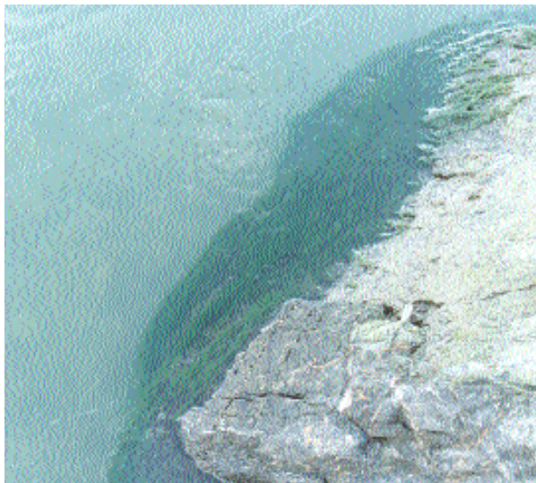
Abbildung 23. Makroalgen-Bewuchs in der Rhone im Spätwinter (März). Bild links oben: Riffle in der Restwasserstrecke von Iles Falcon mit dichtem Kieselalgenbelag und fädigen Grünalgen ( Cladophora sp.) bis zur Uferlinie. Bild links unten: Blockwurf in der Schwallstrecke von Riddes 1 mit dichtem Bewuchs von Cladophora sp., teils über der aktuellen Wasserlinie. Bilder rechts: Schwallstrecke bei Chippis mit Bewuchs der fädigen Grünalge Ulothrix sp. an und teilweise über der aktuellen Wasserlinie (oben); weiter flussaufwärts folgen bei genügend flachem Ufer zuerst eine weitgehend bewuchsfreie Zone und danach ein brauner Streifen mit dichteren Kieselalgenbelägen (unten).
