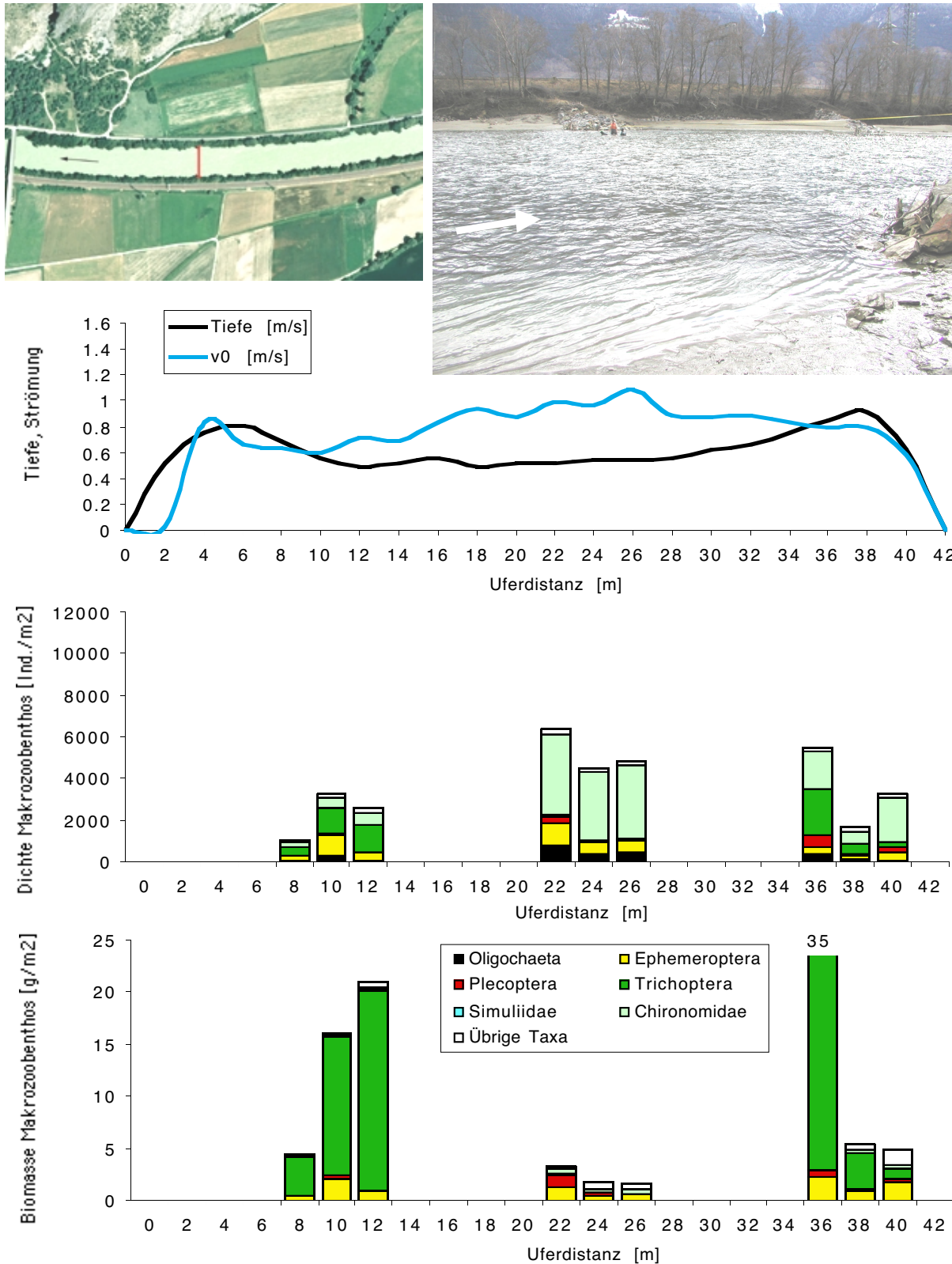
Abbildung 27. Das Makrozoobenthos im Querprofil der Rhone bei Leuk. Von oben nach unten: Luftaufnahme bei hohem Wasserstand im Sommer 1999 oder 2000 mit der Lage des Querprofils (roter Balken) und Ansicht des Profils zum Zeitpunkt der Aufnahmen; Wassertiefen und Oberflächenströmung v_0 über das Profil bei tiefem Abfluss am 26.1.2002; Abundanz (Individuendichte) und Biomasse (Frischgewicht) des Makrozoobenthos in Einzelproben über das Profil am 3.3.2002, aufgeteilt nach den wichtigsten vertretenen, systematischen Gruppen. Darstellungen der Querprofile in Fließrichtung betrachtet. Luftbild: Aufnahme "Swissimage", © Office fédéral de topographie (DV023268).
