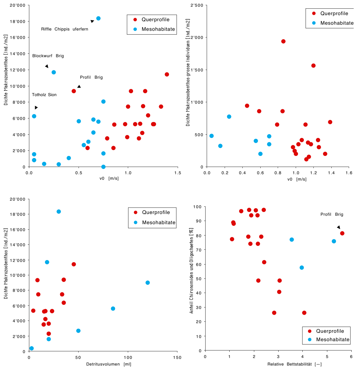
Abbildung 35. Beziehung zwischen abiotischen und biotischen Parametern aus Quersprofilen (Mittel aus drei Einzelwerten) und Mesohabitaten (Einzelwerte) der Rhone im Winter 2002. Die hydraulischen Kennwerte der Oberflächenströmung ( v_0 ) und der relativen Bettstabilität beziehen sich auf den Wasserstand bei Sunk. Dargestellt sind jeweils alle verfügbaren Wertepaare, in der Grafik links unten fehlt ein extrem abweichender Einzelwert ("Ausreisser").
