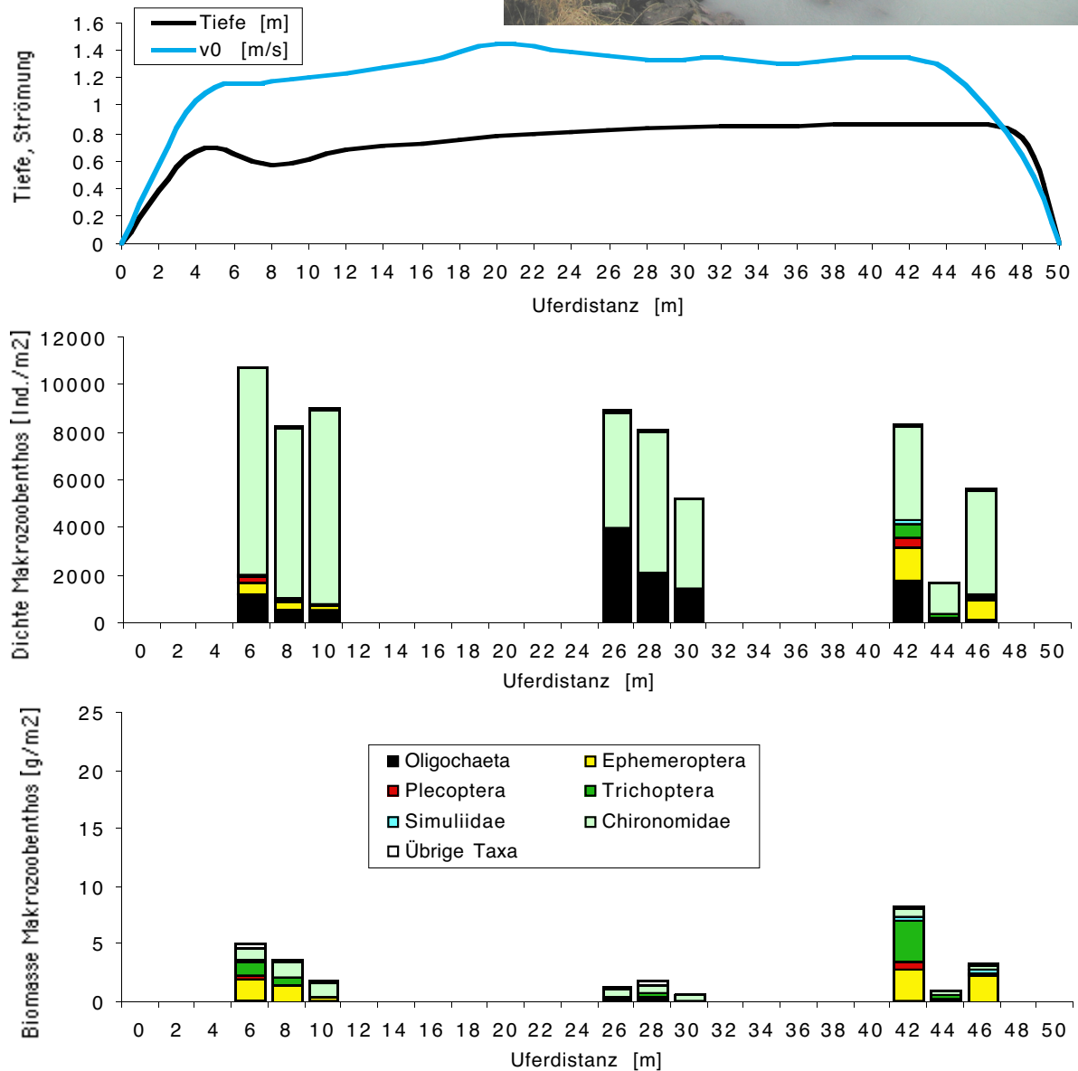
Abbildung 29. Das Makrozoobenthos im Querprofil der Rhone bei Riddes 2. Von oben nach unten: Luftaufnahme bei hohem Wasserstand im Sommer 1999 oder 2000 mit der Lage des Querprofils (roter Balken) und Ansicht des Profils zum Zeitpunkt der Aufnahmen; Wassertiefen und Oberflächenströmung v_0 über das Profil bei tiefem Abfluss am 2.3.2002; Abundanz (Individuendichte) und Biomasse (Frischgewicht) des Makrozoobenthos in Einzelproben über das Profil am 2.3.2002, aufgeteilt nach den wichtigsten vertretenen, systematischen Gruppen. Darstellungen der Querprofile in Fließrichtung betrachtet. Luftbild: Aufnahme "Swissimage", © Office fédéral de topographie (DV023268).
