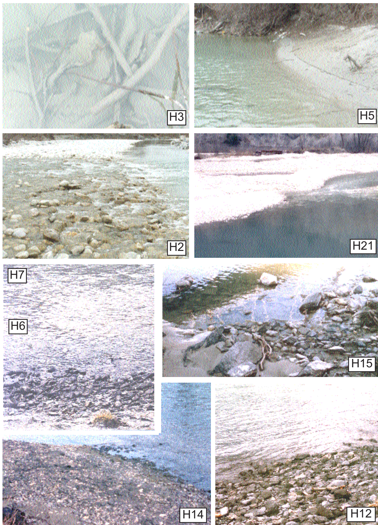
Abbildung 32. Ansichten einiger beprobter Mesohabitate in der Rhone. Von oben links nach unten rechts: Totholz ufernah bei Leuk (H3); Sandbank im Bühnenfeld bei Leuk (H5); Riffle in Flussmitte bei Pfynwald (H2); Kiesbank in Flussmitte bei Iles Falcon (H21, Aufnahme ETEC); Riffle ufernah und -fern bei Chippis (H6 und H7); Grosse Steine bei Sion Vissingen (H15, Aufnahme ETEC); Kiesbank bei Aproz (H14, Aufnahme ETEC); Kiesbank bei Riddes (H12, Aufnahme ETEC).
