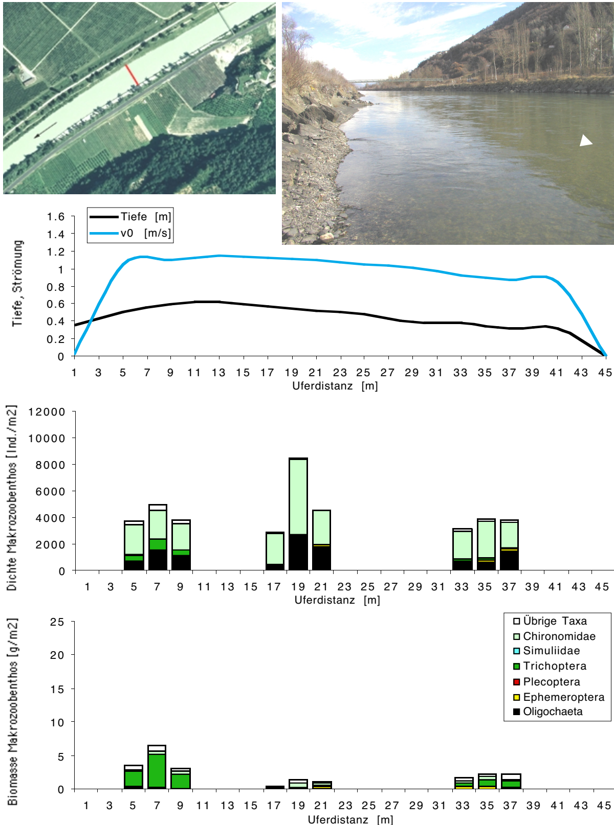
Abbildung 28. Das Makrozoobenthos im Querprofil der Rhone bei Riddes 1. Von oben nach unten: Luftaufnahme bei hohem Wasserstand im Sommer 1999 oder 2000 mit der Lage des Querprofils (roter Balken) und Ansicht des Profils zum Zeitpunkt der Aufnahmen; Wassertiefen und Oberflächenströmung v0 über das Profil bei tiefem Abfluss am 26.1.2002; Abundanz (Individuendichte) und Biomasse (Frischgewicht) des Makrozoobenthos in Einzelproben über das Profil am 3.3.2002, aufgeteilt nach den wichtigsten vertretenen, systematischen Gruppen. Darstellungen der Querprofile in Fließrichtung betrachtet. Luftbild: Aufnahme "Swissimage", © Office fédéral de topographie (DV023268).
