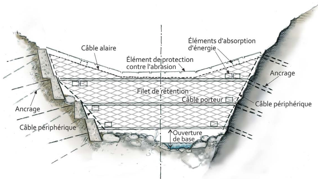
Fig. 1. Vue schématique des composants et de la disposition d'un filet de protection contre les laves torrentielles pour les torrents étroits en forme de V, d'après [12].
