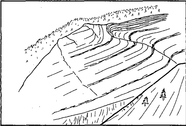
Fig. 13. Paroi de la Schattenfluh vue de la nouvelle route Albinen-Loèche. Faille montrant le « sous-charrriage » au N (droite) des parties inférieures.
