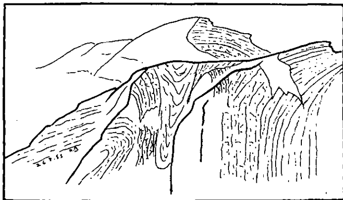
Fig. 17. Synclinal pincé toarcién et domérién. Le Schafberg vu du N, sur l'arête du Torrentborn. En bas à gauche, le noyau de l'anticlinal pliensbachien, puis son enveloppe domérienne (en pointillé) et le synclinal toarcién dont la fermeture est bien visible.
