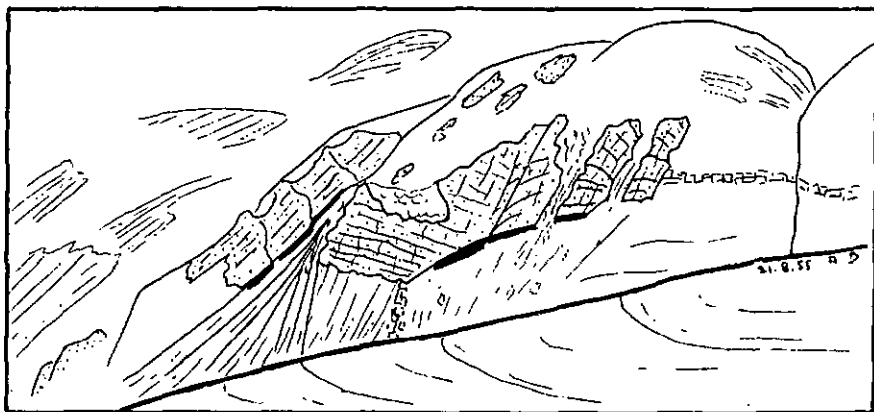
Fig. 19. Dislocations dans le Lotharingien et le Lias inférieur du noyau de l'anticlinal au N de Galm. Paroi dominant le ravin des abreuvoirs au S du Weisssee; au premier plan, crête morainique. En noir, le Lias inférieur; en pointillé, le Lotharingien.
