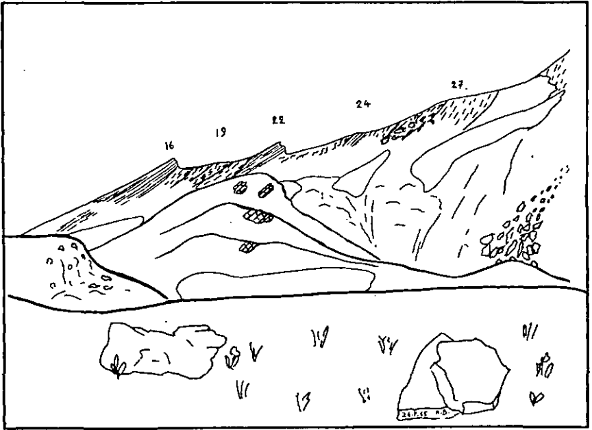
Fig. 15. Arête montant du col de Schnide au Pt. 2806,5, vue de l'E. Au premier plan, le Domérien; alternance sous le col de lames aaléniennes, toarciennes et pliensbachiennes. Les chiffres correspondent à ceux de la coupe donnée à la p. 109.
