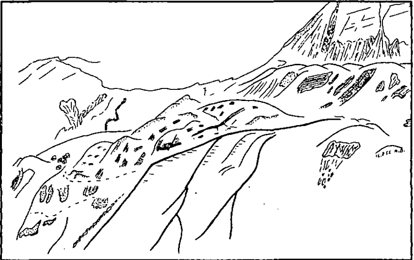
Fig. 18. Pente W du vallon de Bachalp, en amont de Galm et jusqu'au Weisssec. D'un point au NE du Pt. 2401,1. Au fond, l'échancrure du col de Galm. Le Domérien est indiqué par un pointillé lâche, le Pliensbachien par des hachures, le Lotharingien par un pointillé serré; le Lias inférieur est en noir, et le cristallin (à l'extrême droite) en hachures croisées.
