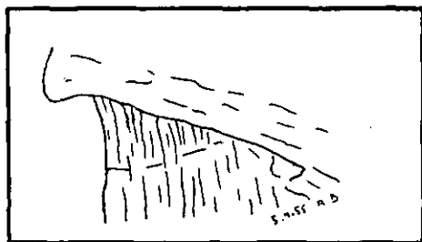
Fig. 9. Discordance entre les gneiss (dessous, N 60 E, verticaux) et la cornicule (dessus, N 110 E ; 30° S). Longueur de l'affleurement 1 m. E de Feschel.
