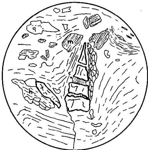
Fig. 2. Fuseau de sphène étiré perpendiculairement à la schistosité actuelle de la roche. Cristaux de quartz ( g ), de hornblende ( h ), de muscovité ( m ) et de calcite ( c ). Grossissement environ 20 diamètres.
