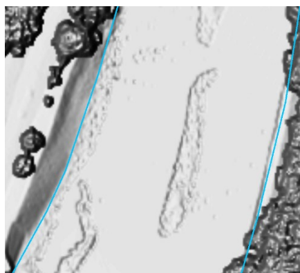
Figure 19: Iles à niveau inférieur par rapport à l'eau
