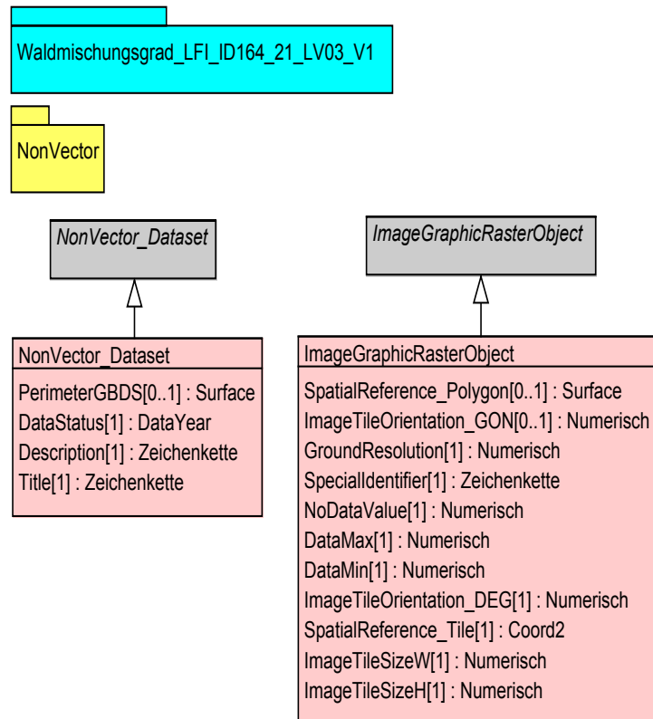
Abbildung 5 UML-Klassendiagramm Rasterdaten
