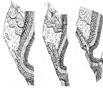
Fig. 3.33 - Formation d'une combe anticlinale 2 (Schaer et al. 1998)
