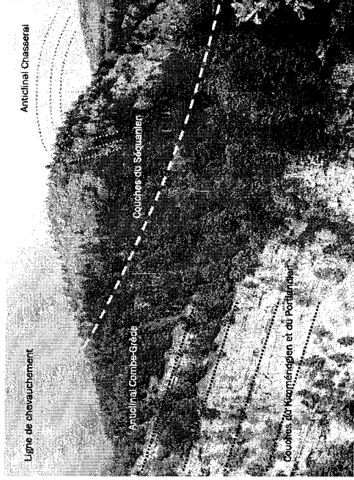
Fig. 4.2 – La zone de chevauchement (Photo : J. von Ballmoos)
