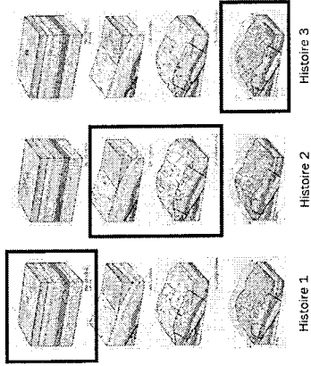
Fig. 3.1 – La schématisation des trois histoires du paysage (modifié d'après ©ISSKA)
