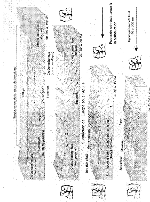
Figure 3.18 - Le plissement des Alpes et du Jura (d'après Schaer et al. 1998)
