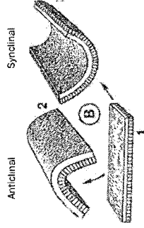
Fig. 3.5 ... Anticlinel et synclinal (d'après Foycault et Raoult 2001)
