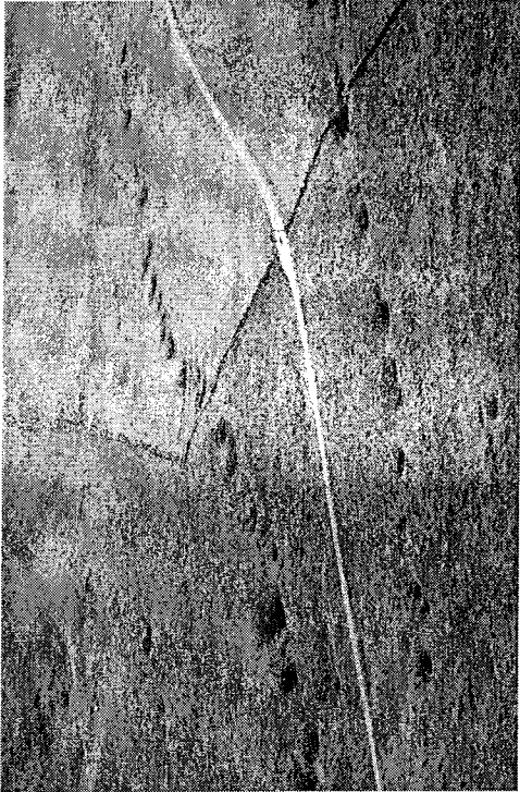
Fig. 3.44 – Alignement de dolines dans la combe anticlinale (Photo : P. von Balmoos)
