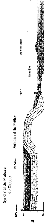
Fig. 3.49 - Coupe géologique du Plateau de Diesse (d'après Schiäl 1971)
