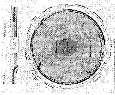
Fig. 3.16 - Structure interne de la Terre (Marchaler 2002)
