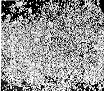
Fig. 3.36 - Sable oolithique d'Abu Dabi (Photo : J. von Ballmoos)
