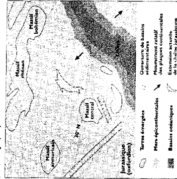
Succèsion paléogéographique du Jura au Jurassique D'après Meunier & Simeyff (1999) et Ziegler (1996).
