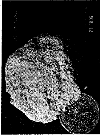
Fig. 3.37 - Calcaire oolithique ( http://www.tcaser.fr/~granderes/bcpst/docs/bp/geo/géologie_petit_chasseral/calcaire_oolithique1.modif1.jpg )
