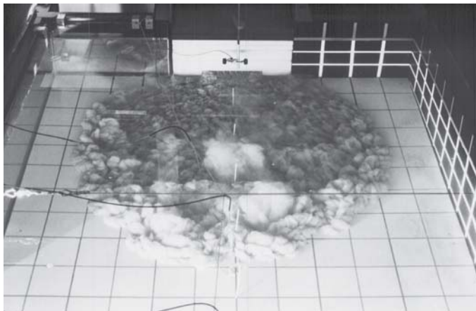
Bild 6. Trübestrom im Labor (Foto: Giovanni De Cesare, EPFL-LCH).
