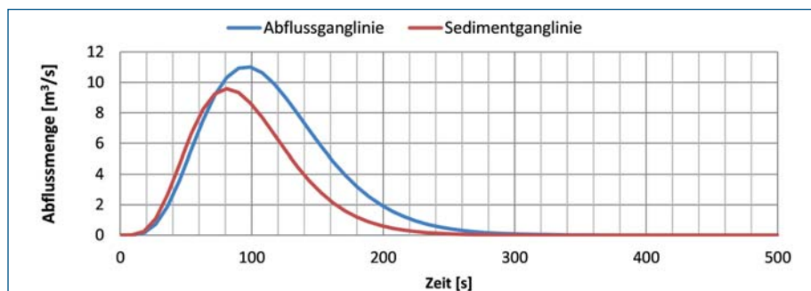
Bild 8. Beispiel eines Zufluss-Szenarios für Wasser ( V = 1009 \text{ m}^3 ) und Sediment ( V_s = 878 \text{ m}^3 ).
