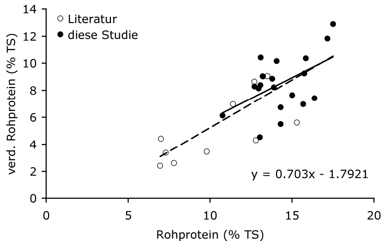
Abb. 7: Rohprotein (% TS) gegen verd. Rohprotein (% TS) aus den eigenen Versuchen und den Literaturdaten beim Elch (aus Tabelle 4)
