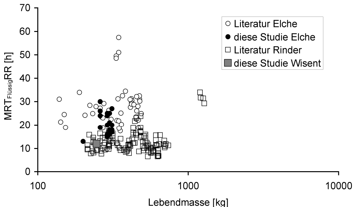
Abb. 10: Lebendmasse gegen MRT_{\text{FlüssigkeitRR}} : Daten von Elchen und Rindern aus der Literatur und von Elchen und der eigenen Studie sowie Literaturdaten von Rindern
