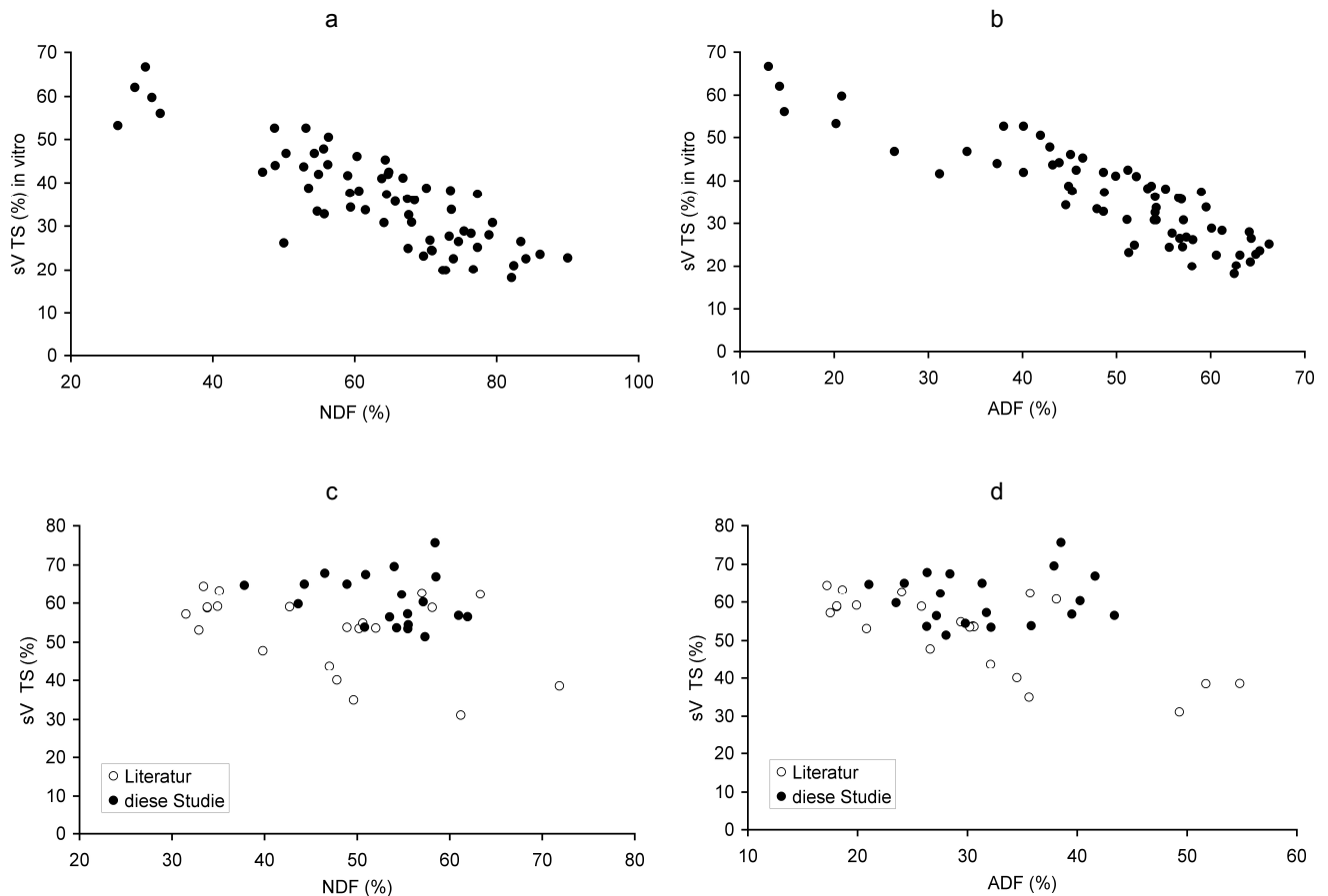
Abb. 5: NDF [%] bzw. ADF [%] der Futterration gegen sV TS [%] aus den eigenen Versuchen und den Literaturdaten für a, b) in vitro mit Elchinokulat (Literaturdaten: HJELJORD et al. 1982, SCHWARTZ et al. 1985, REGELIN et al. 1987, SCHWARTZ et al. 1988c) und c, d) in vivo (Literaturdaten: Für Pellets: SCHWARTZ et al. 1988a; HUBBERT 1987; SCHWARTZ & HUNDERTMARK 1993; SCHWARTZ et al. 1987d; SHOCHAT et al. 1997/ Für Luzerneheu: RENECKER und HUDSON 1990 / Für Grasheu: SCHWARZ & HUNDERTMARK 1993/ Für Zweige: SCHWARTZ et al. 1988e)
