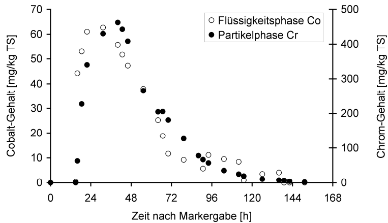
Abb. 2a: Zeitlicher Verlauf der Markerkonzentration im Kot [ \text{mg kg}^{-1} TS] für Cr- und Co des Elches Viola während der Luzerneheu Ration
