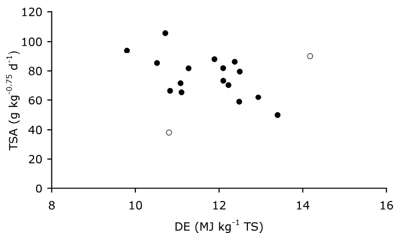
Abb. 4: DE [MJ kg -1 TS] gegen TS-Aufnahme [g kg -0.75 d -1 ] aus den eigenen Versuchen. Ausreißer (offene Symbole): Elch Viola 10.8 DE [MJ kg -1 TS] bei 38.1 [g kg -0.75 d -1 ] auf Luzerneheu und 14.2 DE [MJ kg -1 TS] bei 89.9 [g kg -0.75 d -1 ] auf Luzerne-, Grasheu
