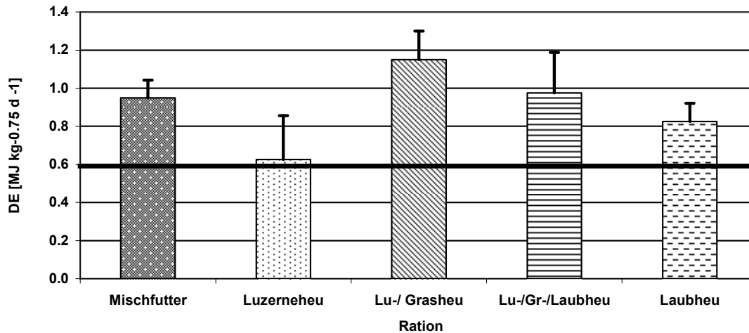
Abb. 14: Aufnahme an verdaulicher Energie (DE) bei den verschiedenen Futterrationen im Vergleich zum von Schwartz et al. (1988a) ermittelten Bedarf (durchgezogene Linie)
