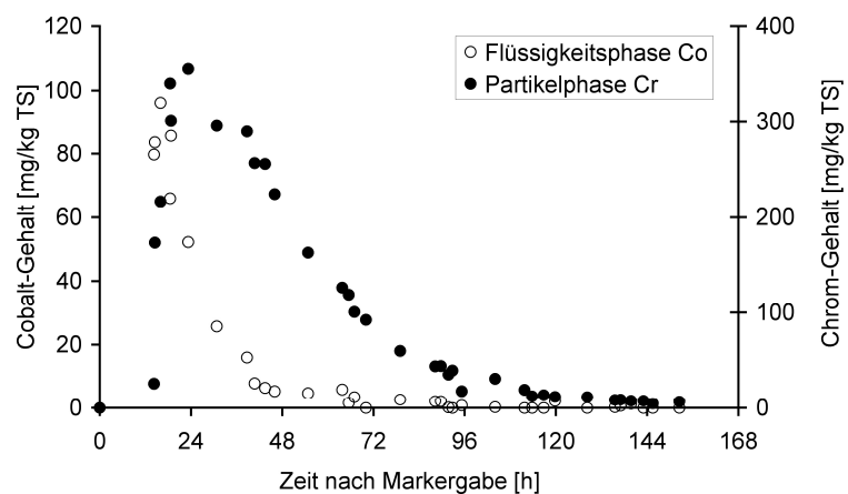
Abb. 2b: Zeitlicher Verlauf der Markerkonzentration im Kot [ \text{mg kg}^{-1} TS] für Cr- und Co des Wisents Luisa während der Grasheu Ration
