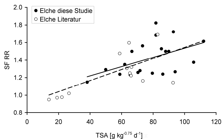
Abb. 12: TS-Aufnahme [g kg -0.75 d -1 ] gegen Selektivitäts-Faktor [h] des RR aus den Daten der eigenen Studie und der Literaturdaten
