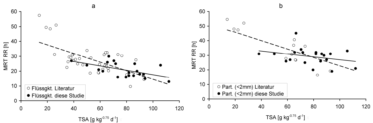
Abb. 9: TS-Aufnahme [g kg -0.75 d -1 ] gegen die Mittlere Retentionszeit im Retikulum [h] aus der eigenen Studie verglichen mit Literaturdaten von Elchen für a) Flüssigkeit und b) Partikel [Literaturdaten für MRT Flüssigkeit RR: RENECKER und HUDSON (1990); HJELJORD et al. (1982); SCHWARZ et al. (1988); HUBBERT (1987); LECHNER et al. (2010); Literaturdaten für MRT Partikel RR: RENECKER und HUDSON (1990), LECHNER et al. (2010)]
