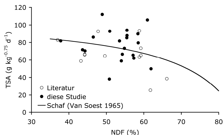
Abb. 3: NDF [%] gegen TS-Aufnahme [g kg -0.75 d -1 ] aus den eigenen Versuchen und den Literaturdaten (aus der Sammlung von Meyer et al. 2010)
