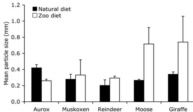
Abb. 13: Vergleich der Kotpartikelgrösse bei Wildwiederkäuern (Aurochse, Moschusochse, Rentier, Elch, Giraffe) in Menschenobhut und in freier Wildbahn aus LECHNER et al. (2010)
