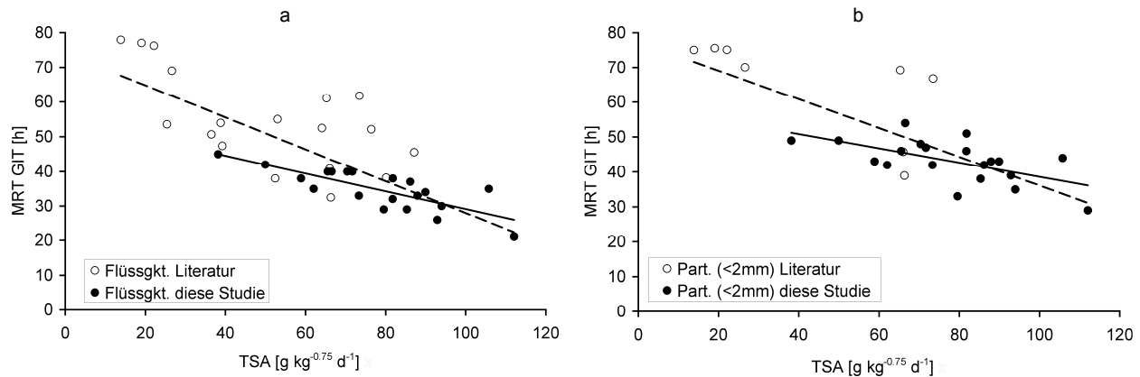
Abb. 8: TS-Aufnahme [ g\ kg^{-0.75}\ d^{-1} ] gegen MRT_{GIT} [h] aus der eigenen Studie verglichen mit Literaturdaten von Elchen für a) Flüssigkeit und b) Partikel
