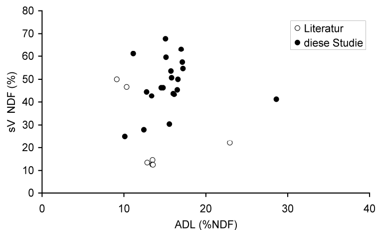
Abb. 6: ADL [%] der Futtration gegen sV NDF [%] aus den eigenen Versuchen und den Literaturdaten beim Elch (aus Tabelle 4)
